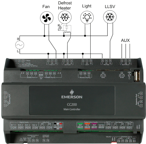
Output Wiring
